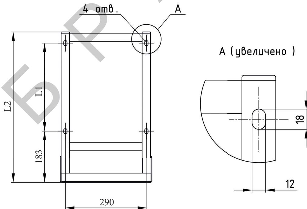
Рисунок 1 – Общий вид изделия в сборе
