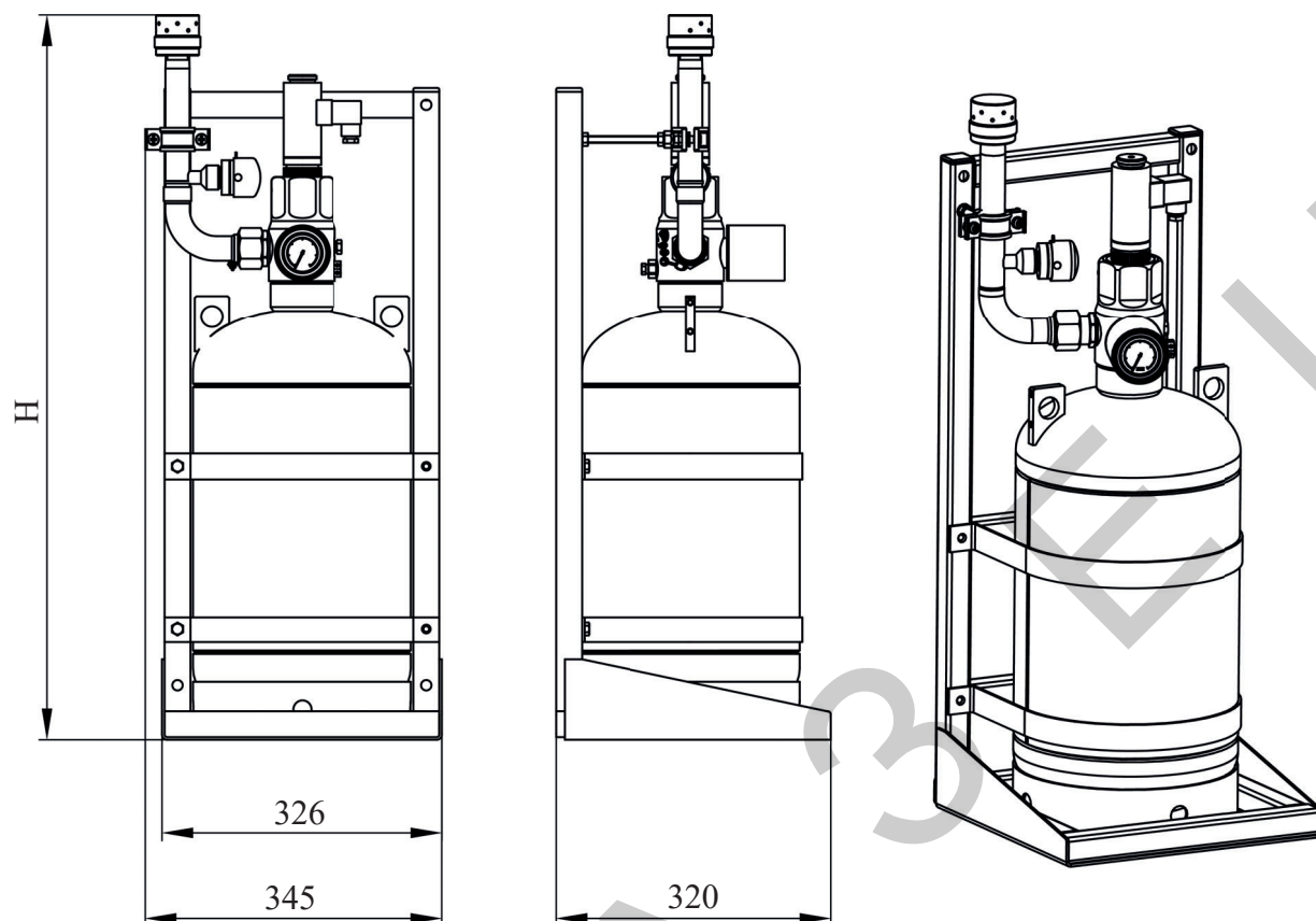
Рисунок 1 – Общий вид изделия в сборе
