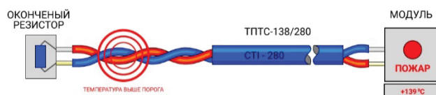
Рис. 2. Режим ПОЖАР
